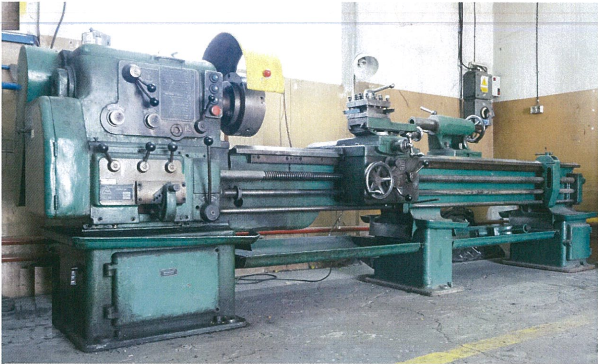
Tokarka TUJ 48
